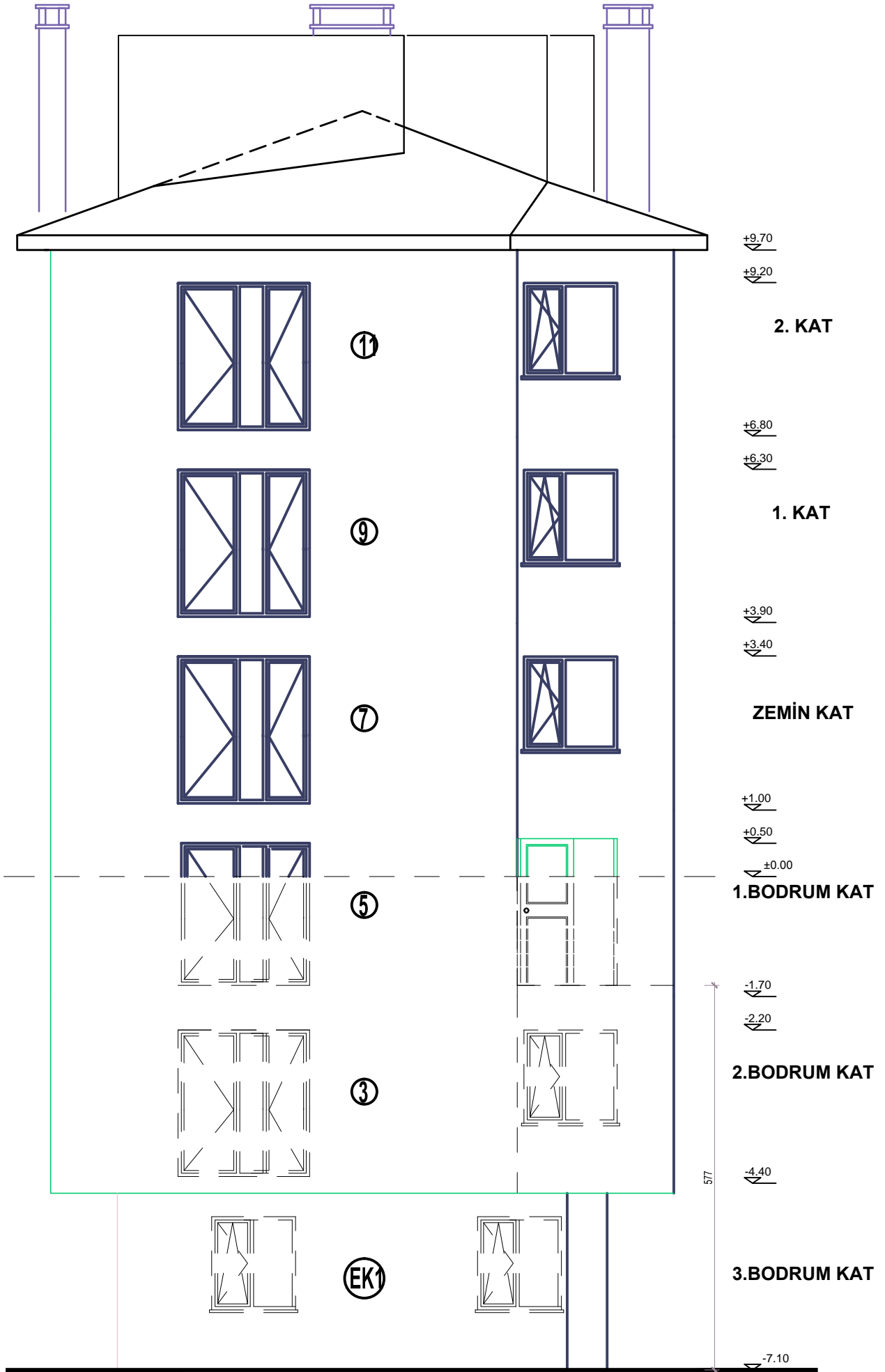
ARKA CEPHE Ö:1/50
